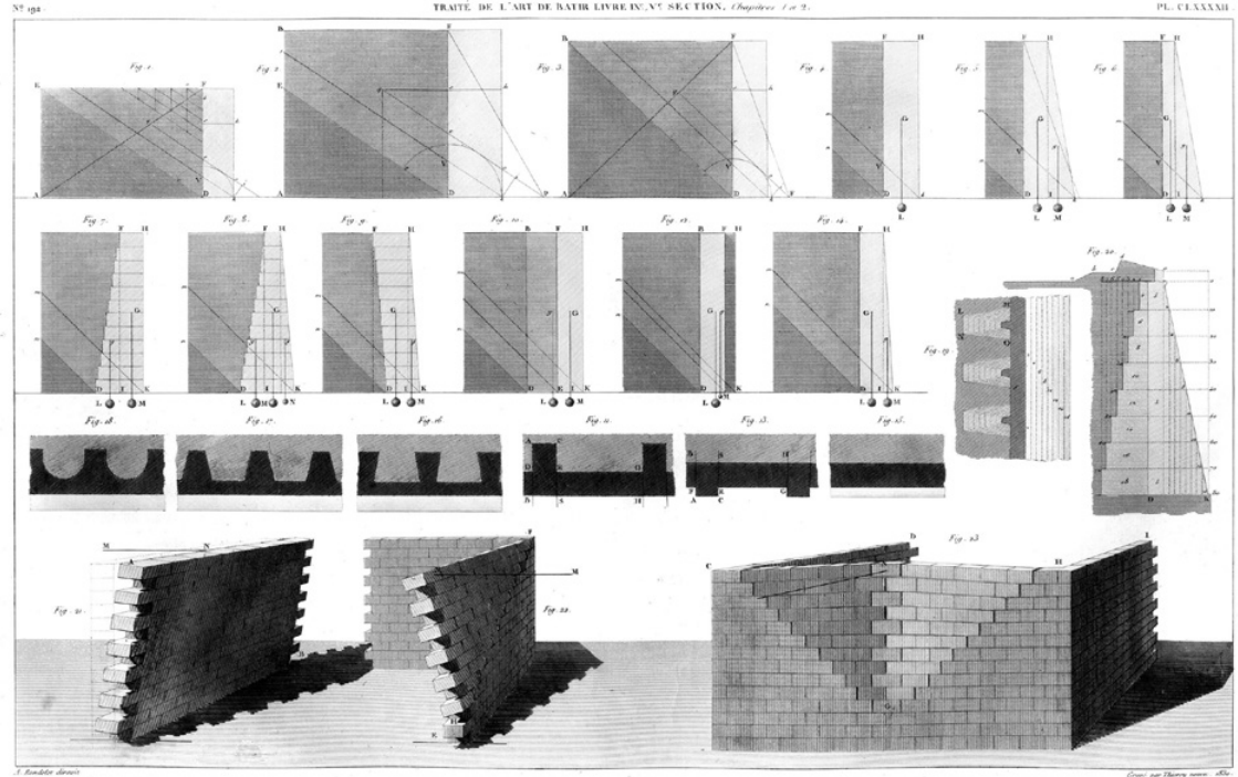
Fig. 2. Jean Baptiste Rondelet, 1814, Traité de l'art de bâtir, Parigi, Libro IX, Tomo V, Tavola CLXXXII.
